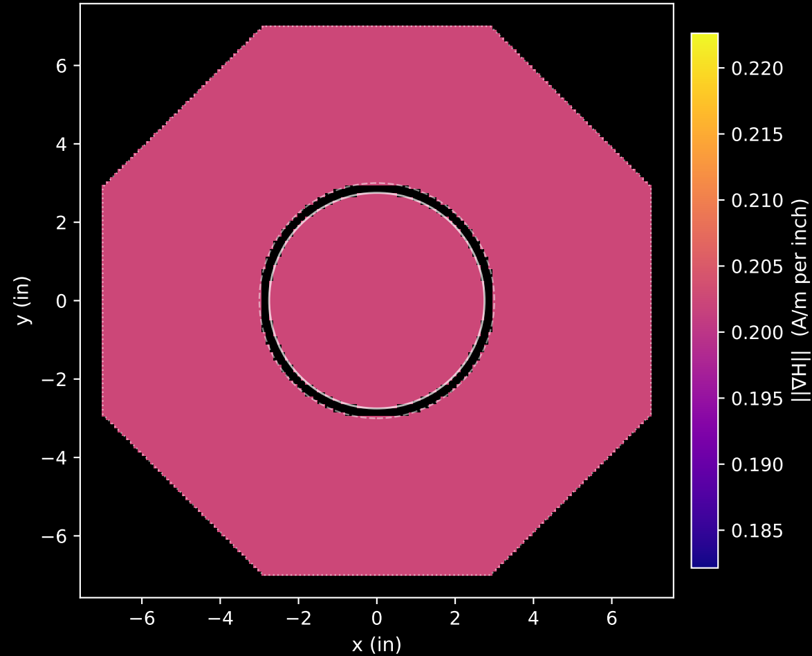
Gradient magnitude
